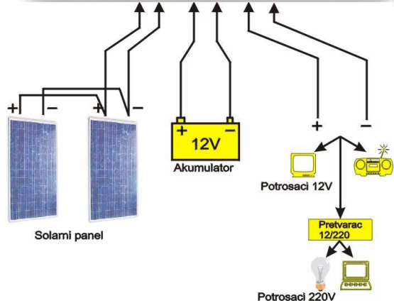
Šema veze regulatora sa panelima, akumulatorom i potrošačima
